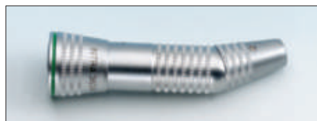
Underdel 3624 N Nedväxlad 4:1
