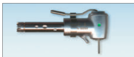
Kirurgihuvud INTRA C3 Sprayanslutning för extern kylning genom fast monterat sprayrör samt intern borkkylning enligt Kirschner & Meyer. Nedväxlat 3:1 Roterande
